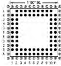
68 Pins – Footprint #11032-ZIF
