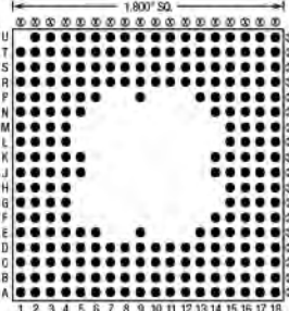
241 Pins – Footprint #18032-ZIF
