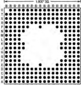
241 Pins – Footprint #18032-ZIF
