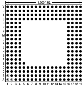
238 Pins – Footprint #19004-ZIF
