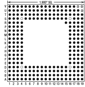
238 Pins – Footprint #19007-ZIF
